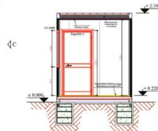
Coupe de principe 1-1
