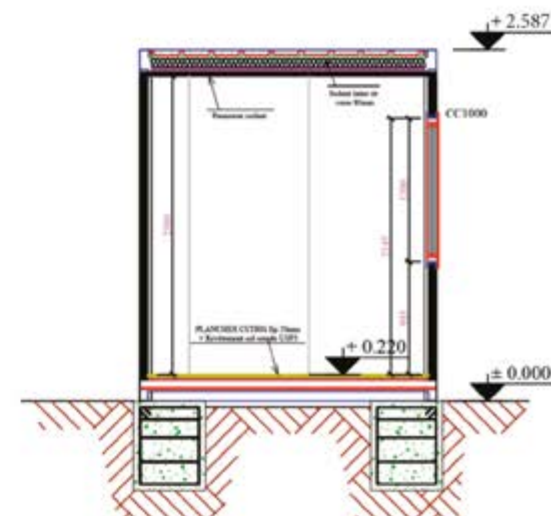
Coupe de principe 1-1
